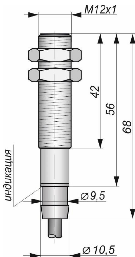
Габаритный чертеж
